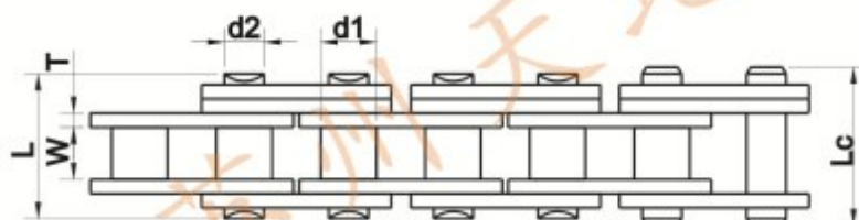
T型 T type
