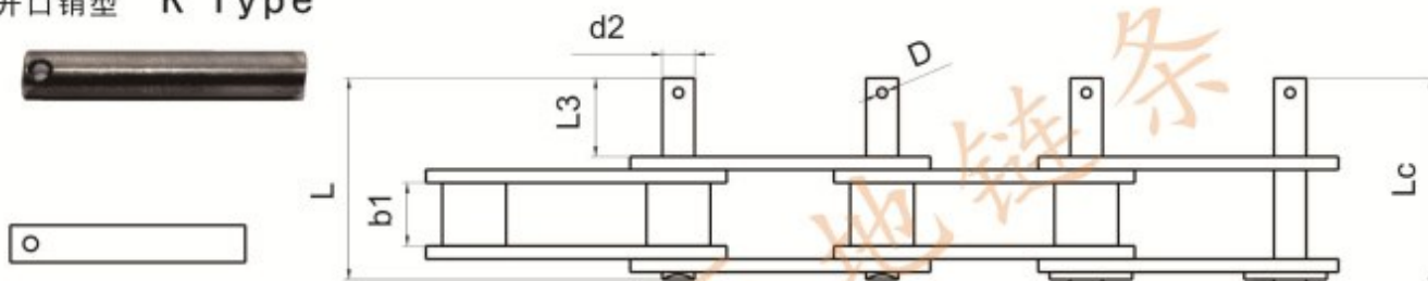
开口销型 K Type
