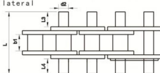
双侧长销 E1 Bilateral
