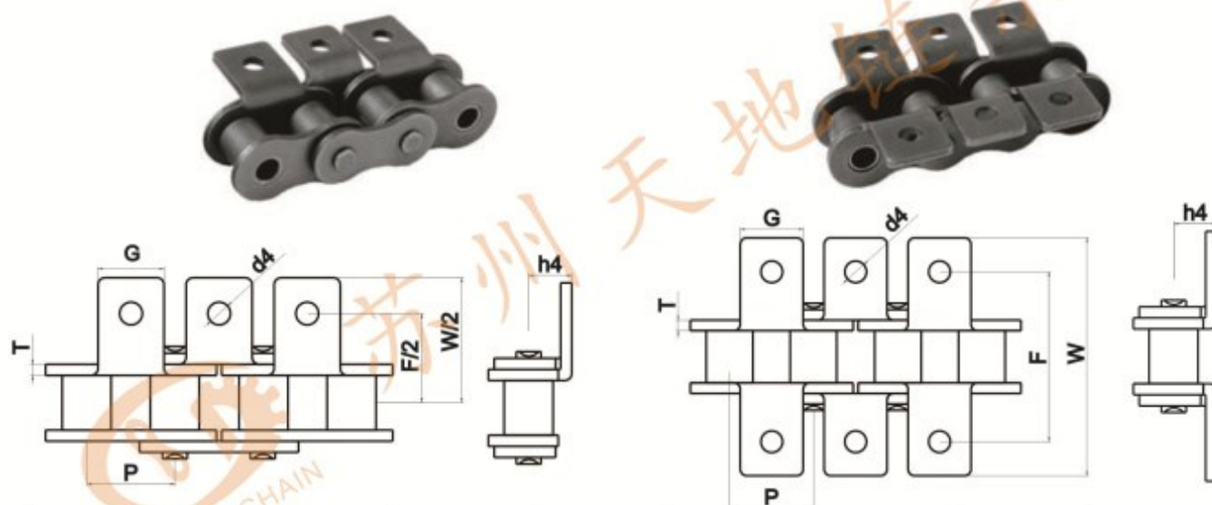
双侧 K-1 Bilateral
