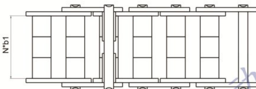
三排加宽链 Dilated triplex chain
