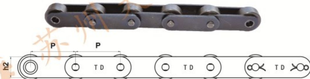
直板型 C straight side
