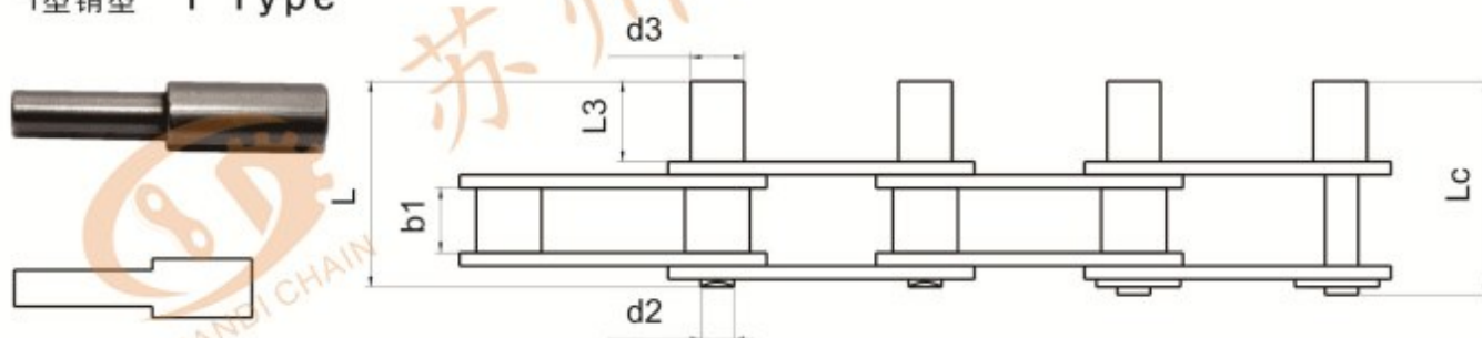
T型销型 T Type
