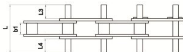
双侧长销 E1 Bilateral
