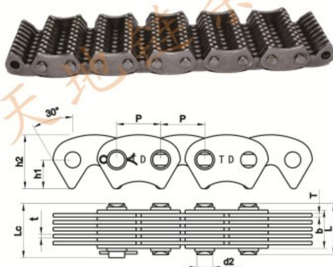
外导式 Side guide
